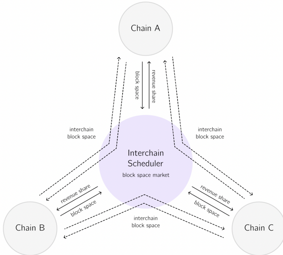
圖 8: 調度器為鏈間區塊空間創建了一個協議內市場，允許鏈指定允許的 MEV。與其他只與驗證者分享收入的解決方案不同，調度器也與消費鏈分享收入。
